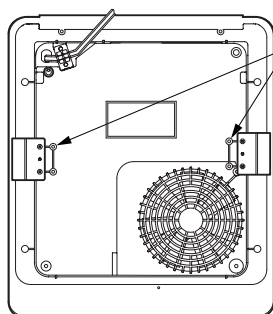
左右固定用バネ 取付部 ※外側の取付穴 を使用
