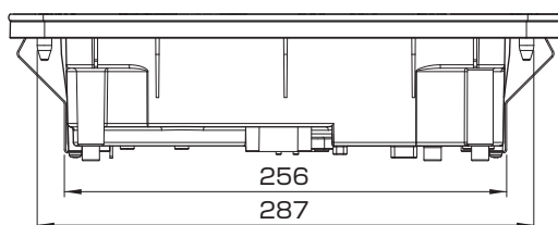
正面図
