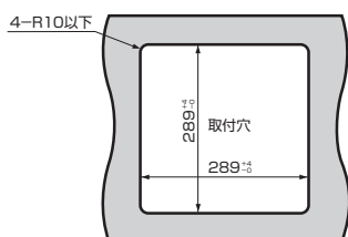
本体取付穴
