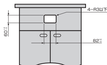
コントロールボックス 取付穴
