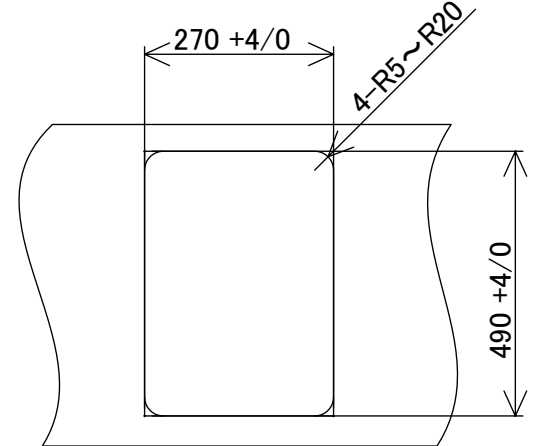
取付開口寸法
