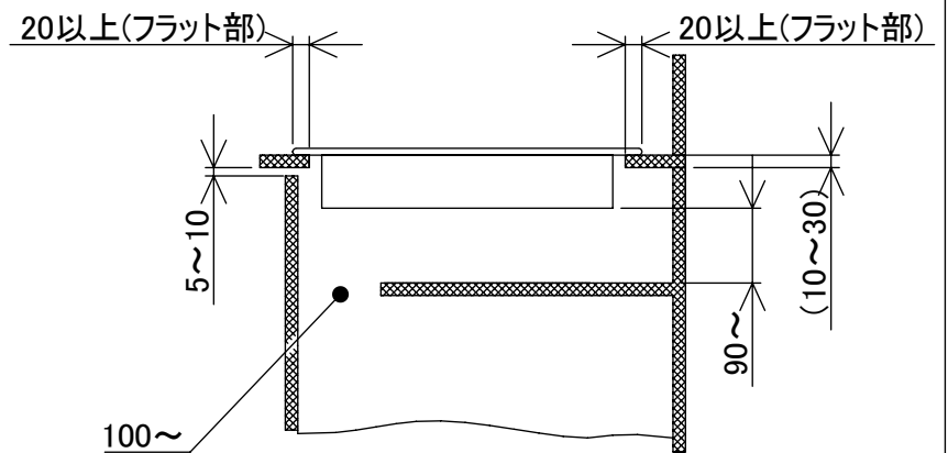
取付側面
