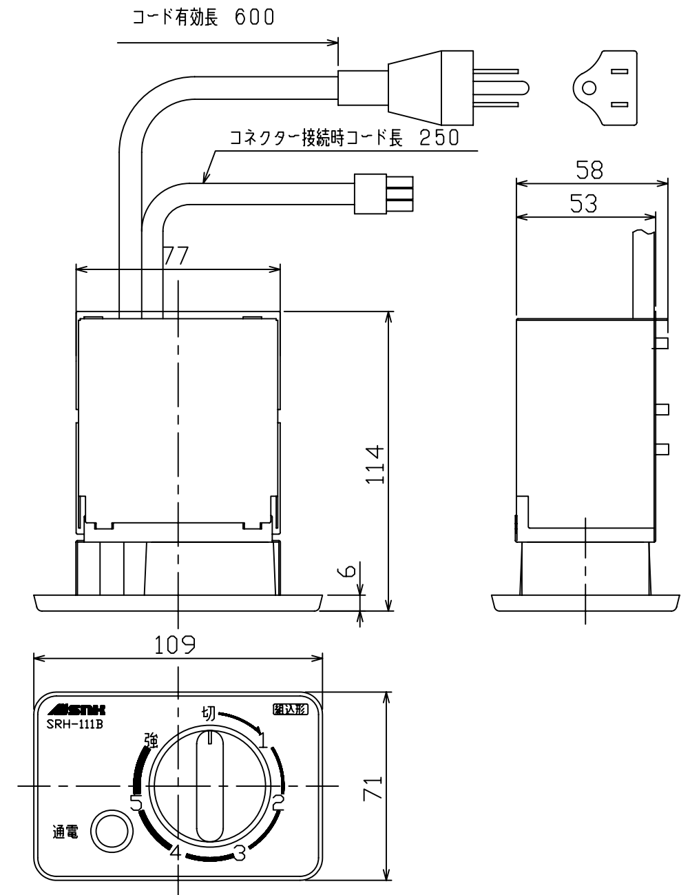
熱量調節器
