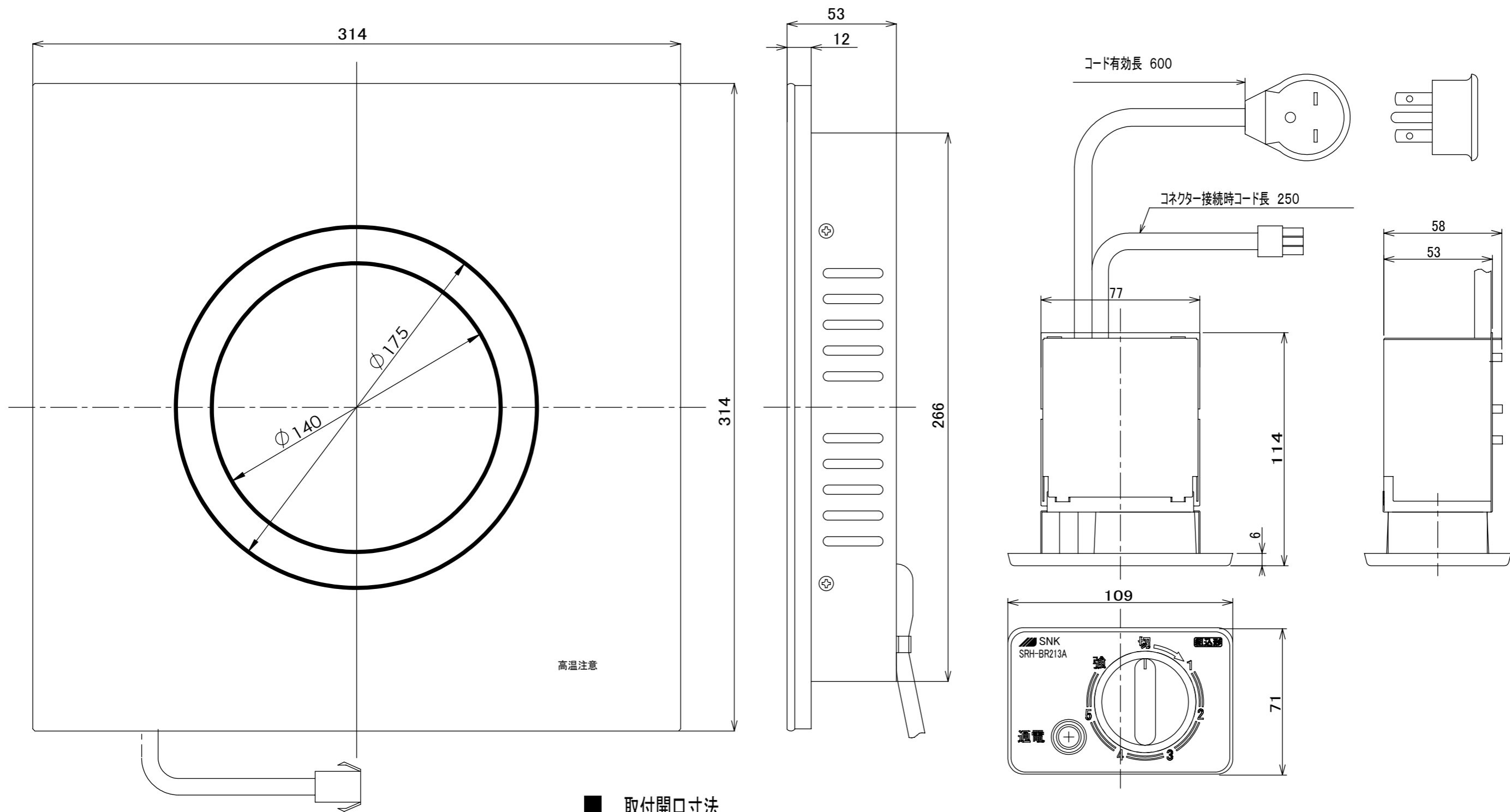
熱量調節器
