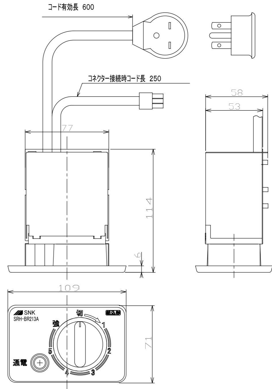
熱量調節器
